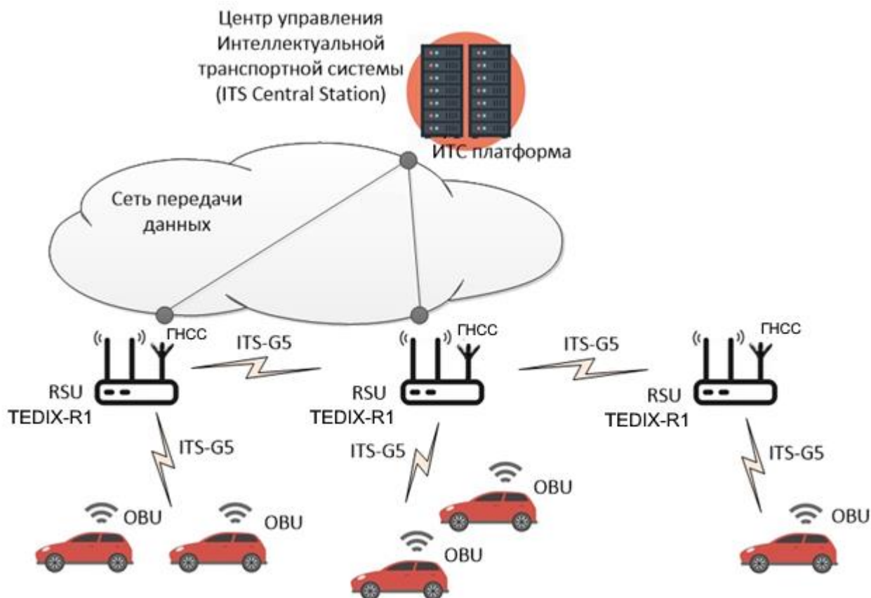
Рисунок 3.7 – Взаимодействие OBU TEDIX – V1 с RSU TEDIX-R1
