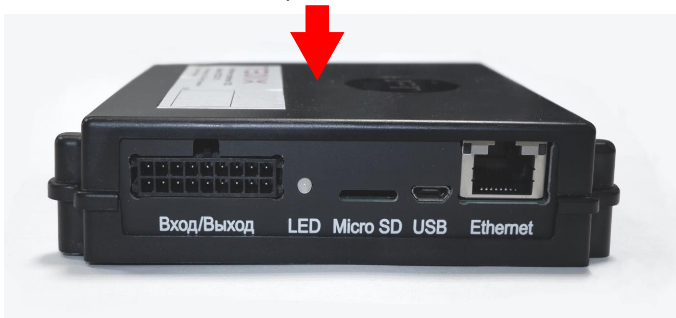
Рисунок 4.1. Ориентация TEDIX-V1 при установке в транспортном средстве
